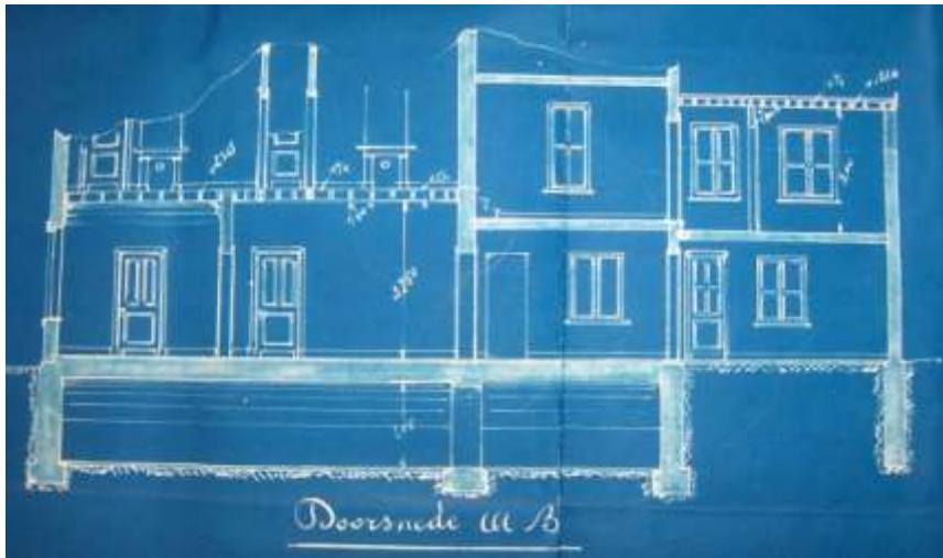
Dwarsdoorsnede huis Boschstraat 30
